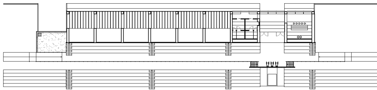
Pianta piano primo locali sotto tribune - Bar e servizi igienici
